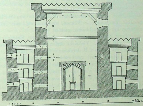
Abb. 122. Querschnitt des Tempels.
