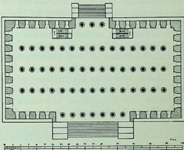
Abb. 119. Libanonwaldhaus, Grundriss.
