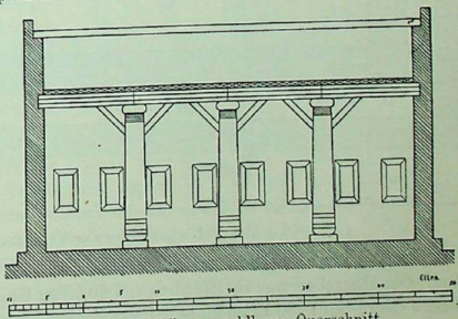
Abb. 120. Libanonwaldhaus, Querschnitt.
