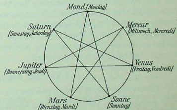
Abb. 82. Verteilung der Wochentage nach dem Heptagramm.
