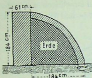
Abb. 228. Mauer von Gezer, Querschnitt.
