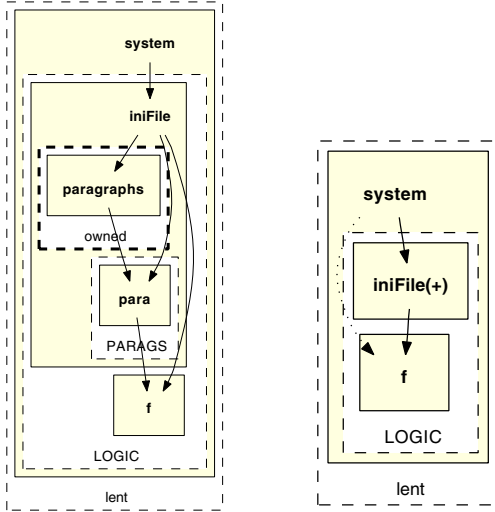
(b) Expanded OOG.
